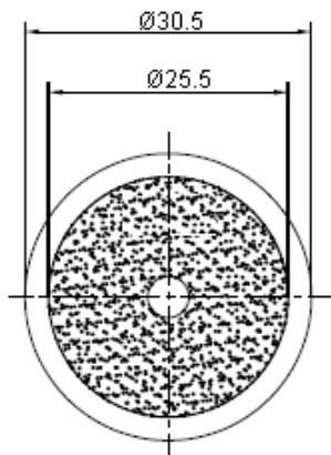
Dimensions : Millimetres
