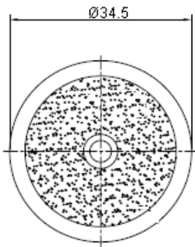
Dimensions : Millimetres
